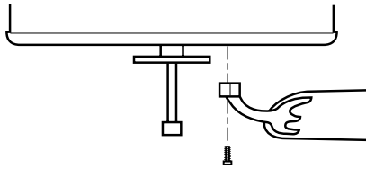
Figura 7d - Fixando os prendedores de pás ao cubo do conjunto do ventilador
