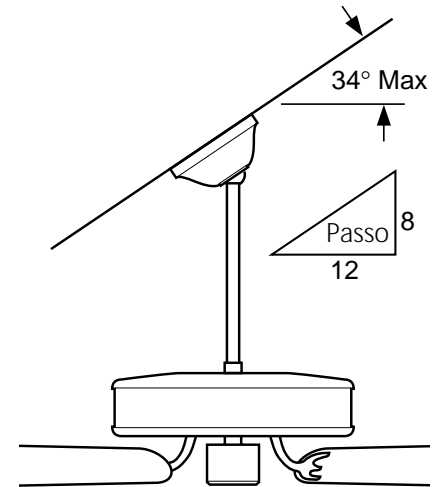
Figura 1c - Montagem em ângulo
