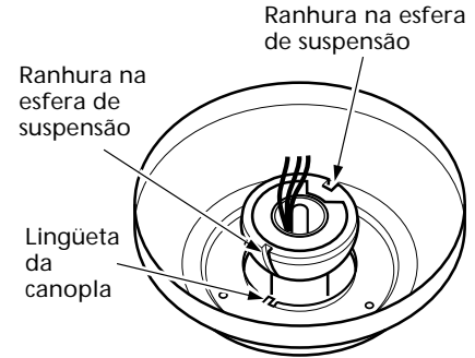
Figura 6b - Lingüetas da canopla e ranhuras na esfera de suspensão
