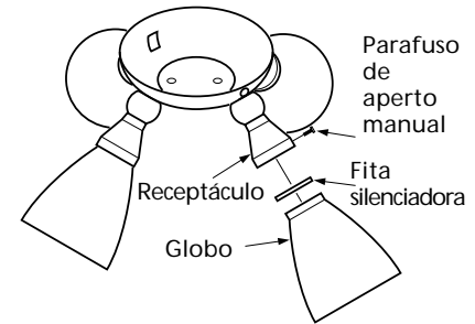
Figura 9d - Kits de iluminação multi-lâmpadas
